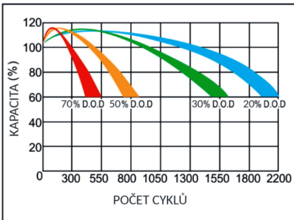
Cyklická odolnost v závislosti na hloubce vybití řada GOOWEI ENERGY - DEEP CYCLE
